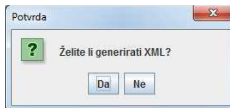
Slika 6.23: Generiranje datoteka
