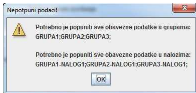
Slika 6.24: Nepotpuni podaci
